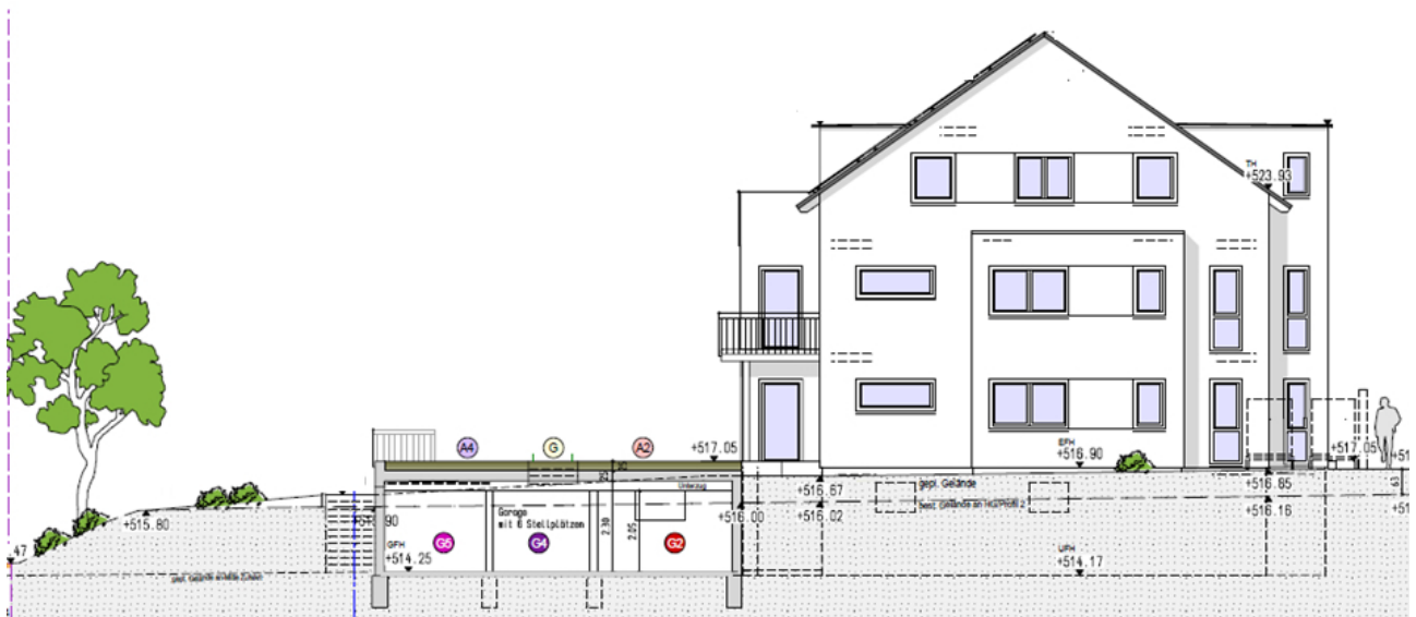
Nordost Ansicht
