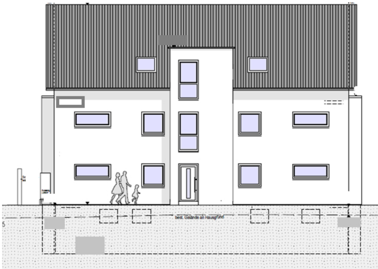
Nordwest Ansicht
