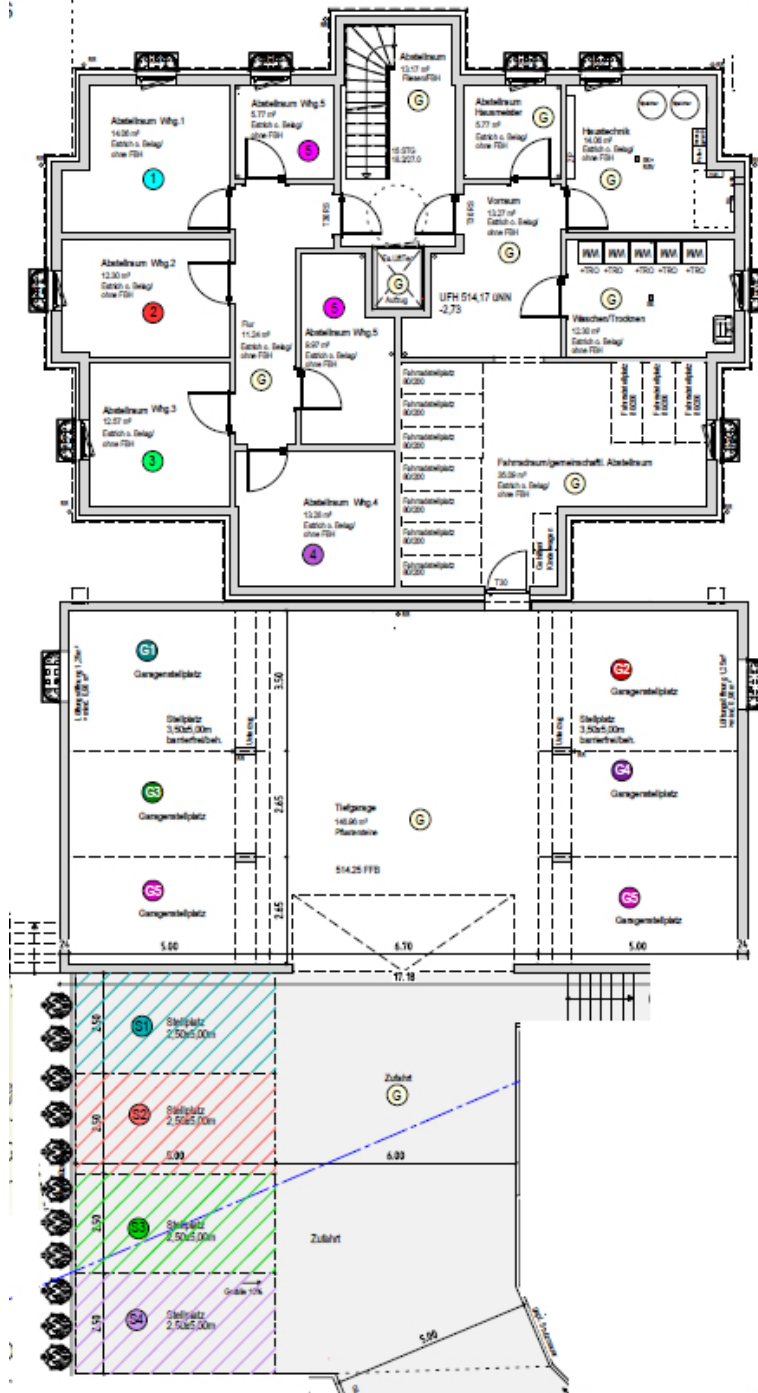
Grundriss UG
