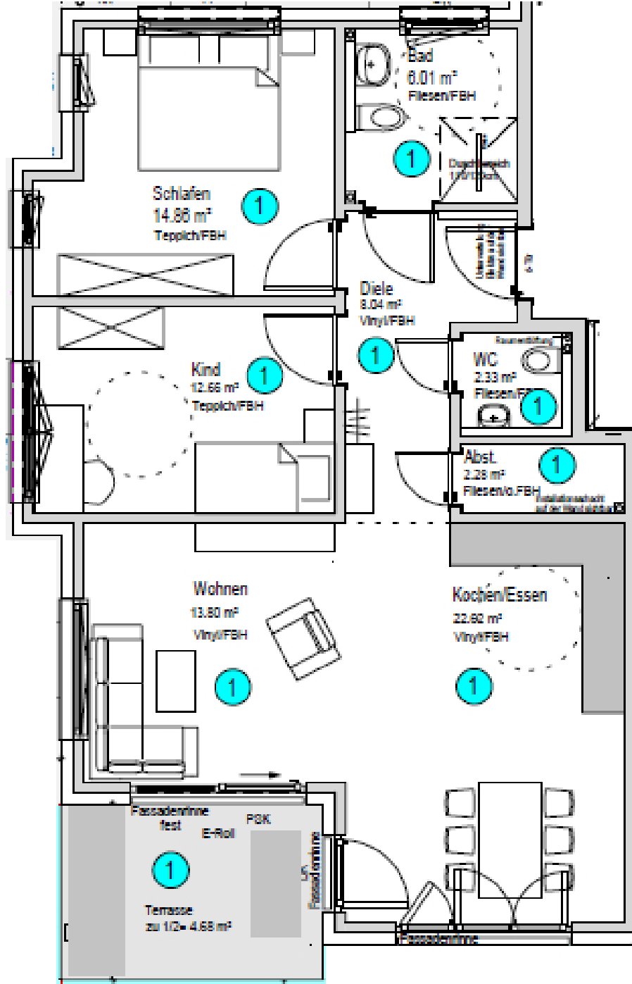
Grundriss Wohnung 1 EG rechts
